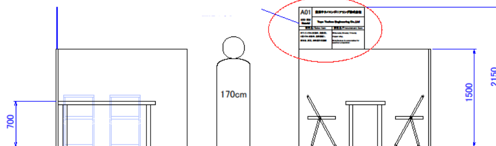
洽谈区域图
